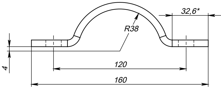
Поз.4 (Полухомут) развертка
